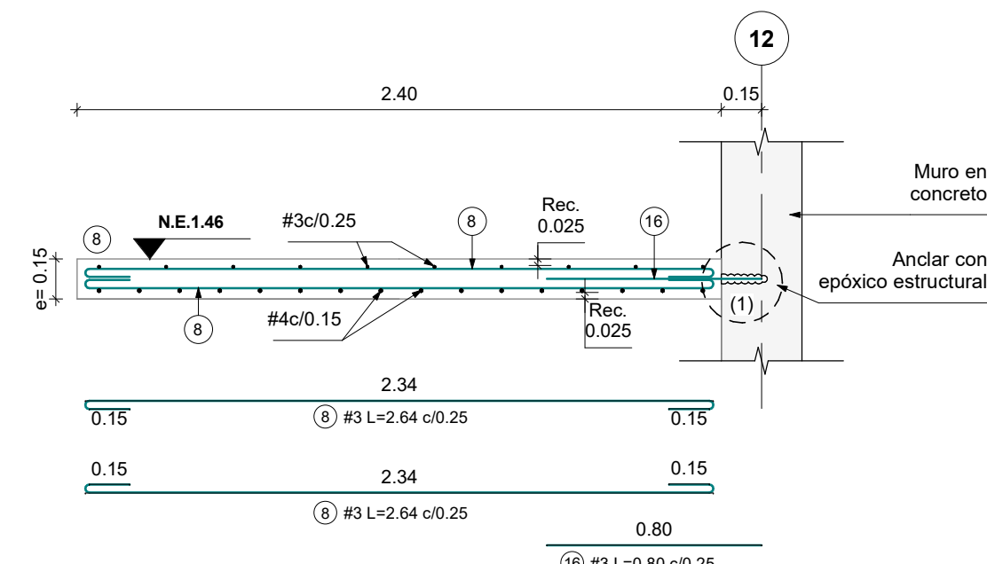
CORTE E-3 Escala 1 : 25
