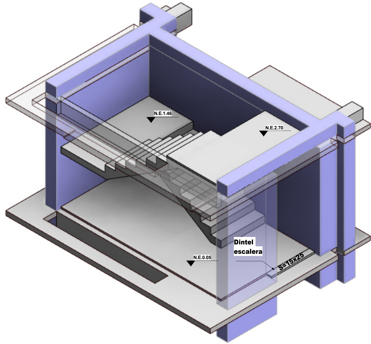
3D ESCALERA TIPO 2 DE PISO 1 A PISO 2 Sin escala
