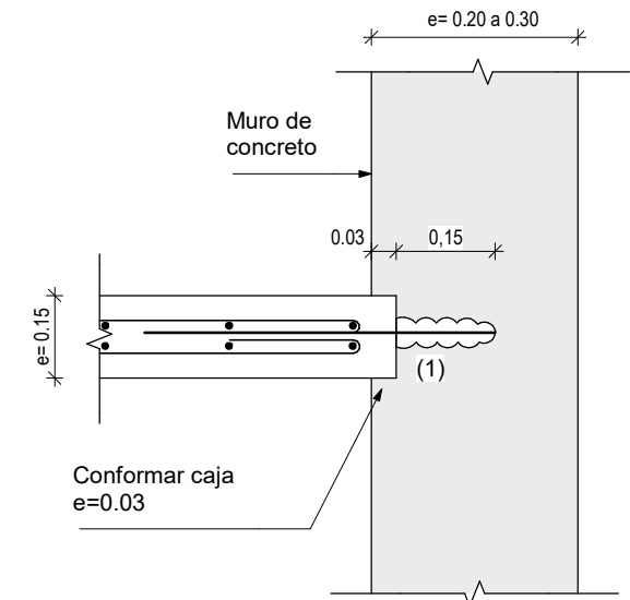
DETALLE 1 Escala 1 : 10
