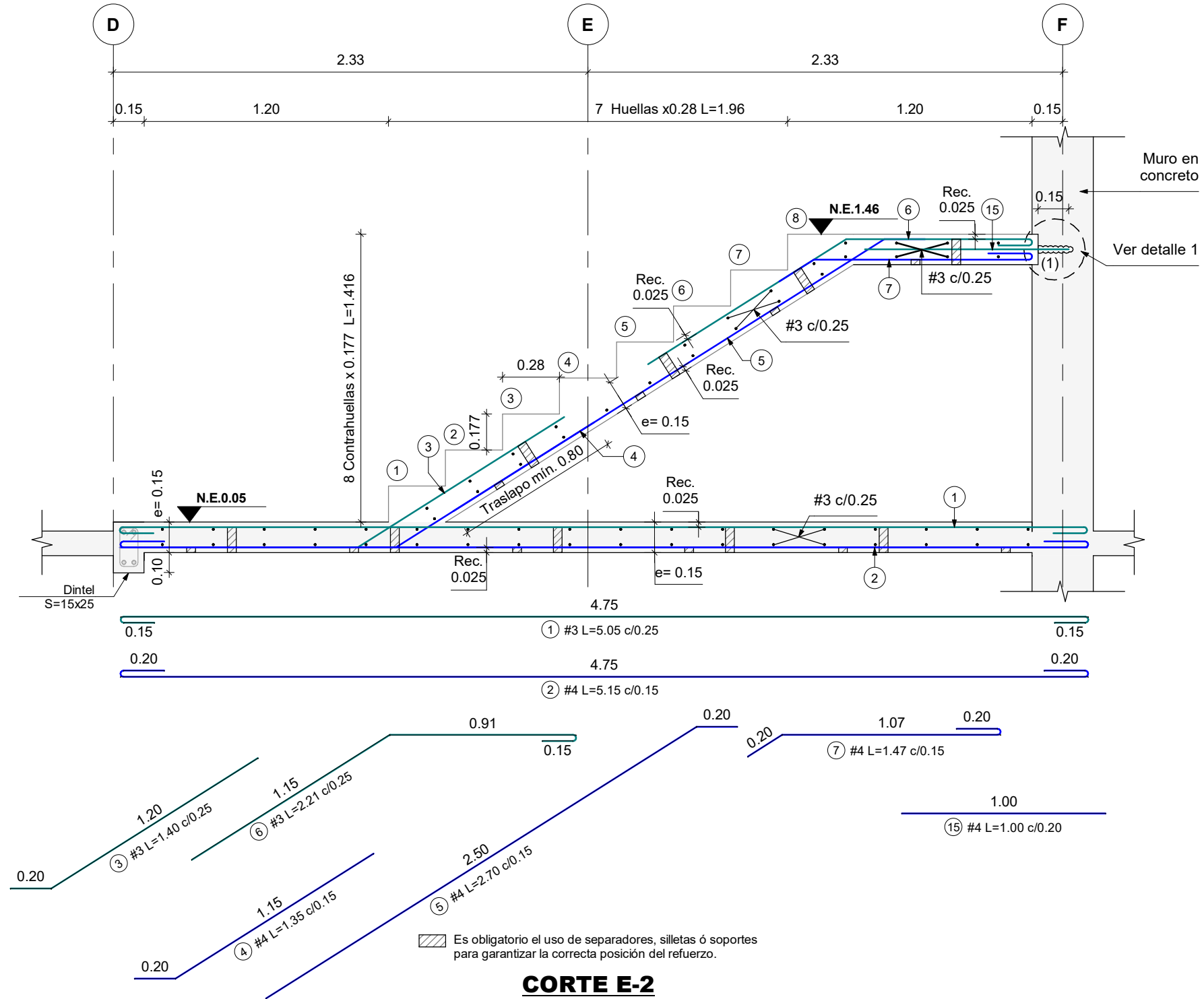
CORTE E-2 Escala 1 : 25
