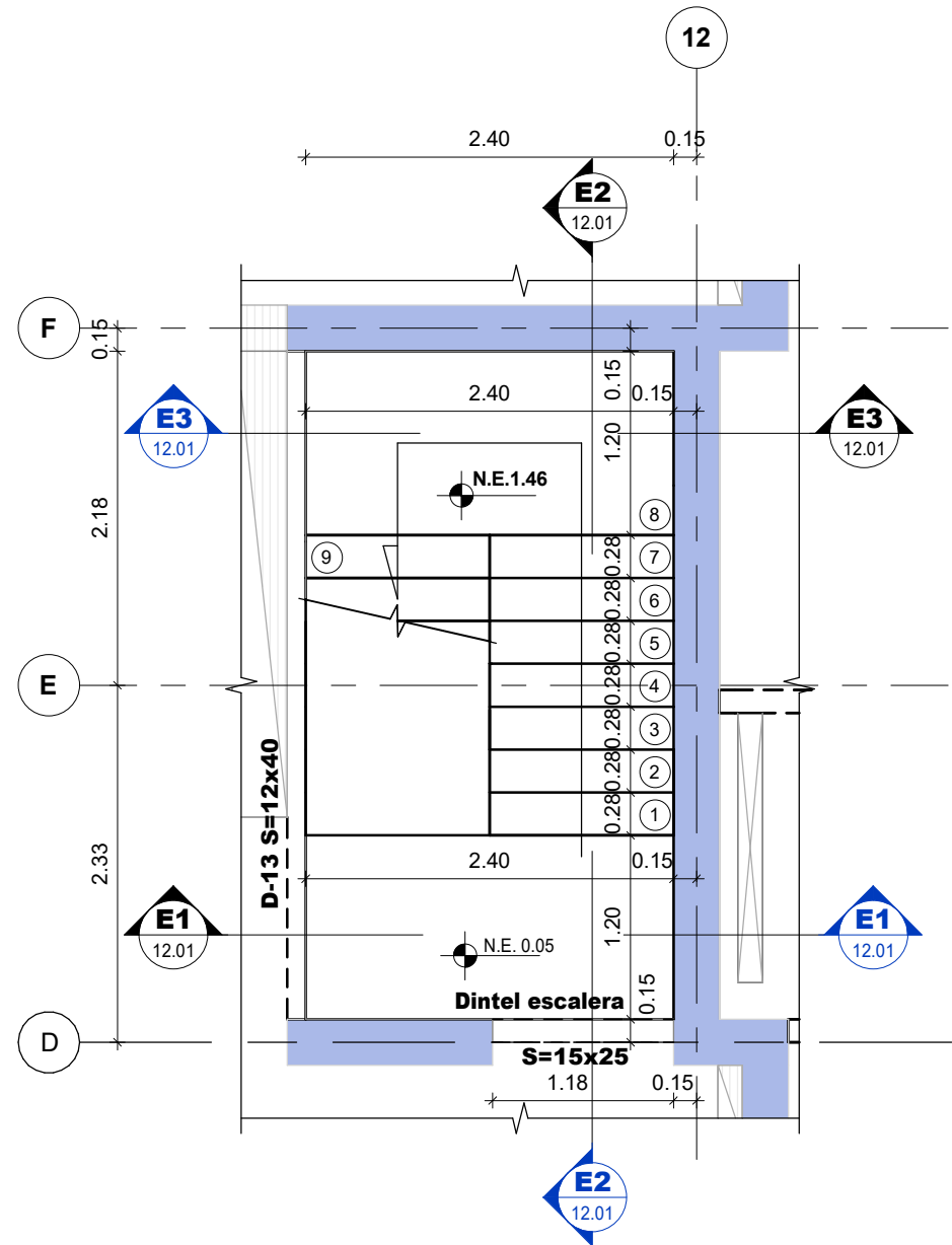
PLANTA ARRANQUE ESCALERA TIPO 2 (PISO 1 A 2) Escala 1 : 50
