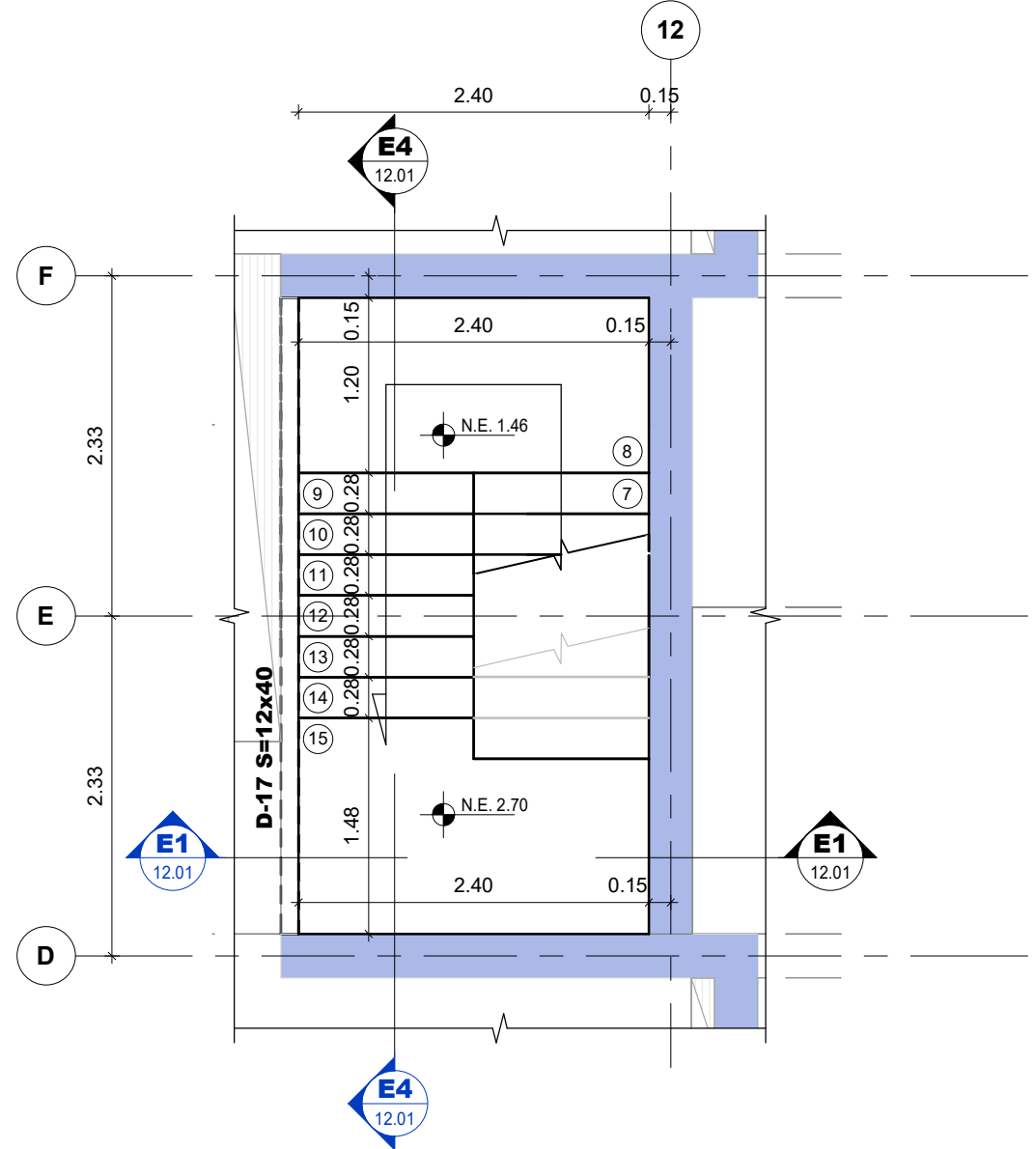
PLANTA LLEGADA ESCALERA TIPO 2 (PISO 1 A 2) Escala 1 : 50
